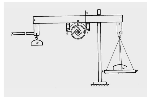
Schéma du dispositif d'essais de G.A.Hirn (1854)
